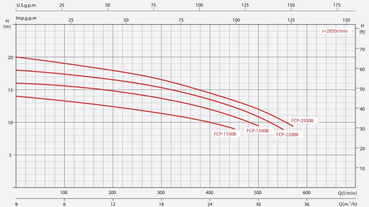
GRÁFICO DE DESEMPEÑO A n=2850 r/min
